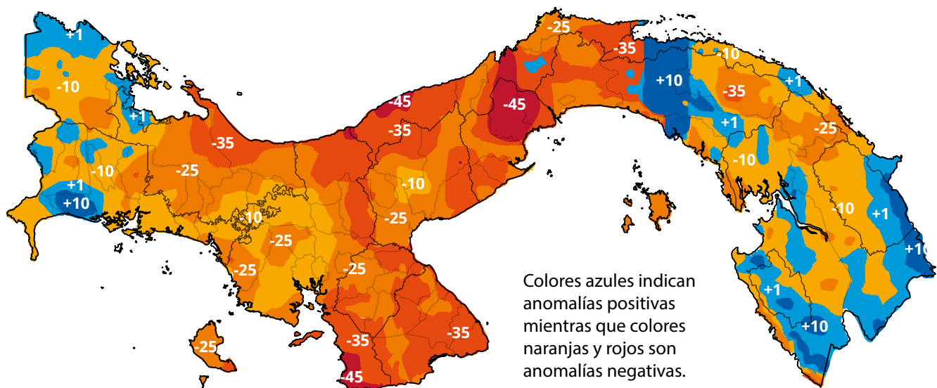
Figura 27. Déficit de lluvia observada entre enero y julio de 2015 en Panamá durante el fenómeno de El Niño, en comparación con la media mensual histórica del periodo 1981-2014.
